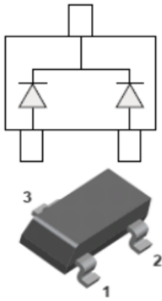
SOT-323
